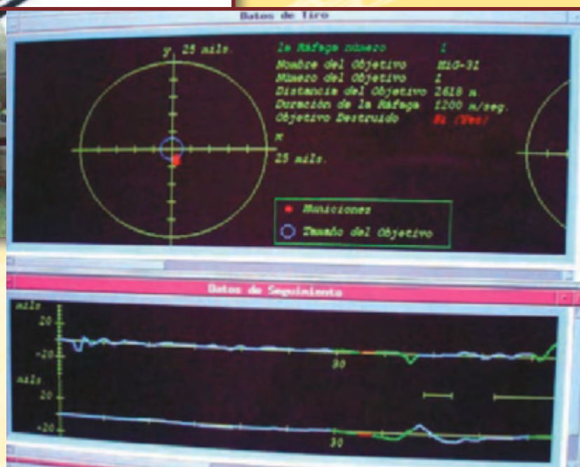
Imagen superior cañón 35/90 GDF 005.
